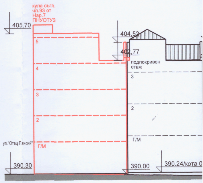
СИЛУЕТ ПО ул. КЪКРИНА М 1:200
