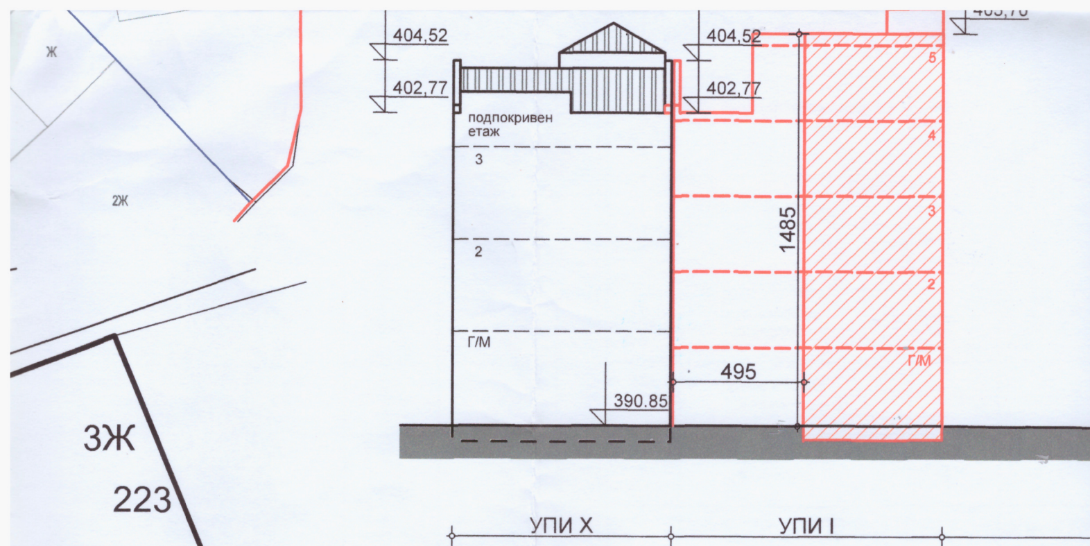
СИЛУЕТ- РАЗРЕЗ 1-1 М 1:200
