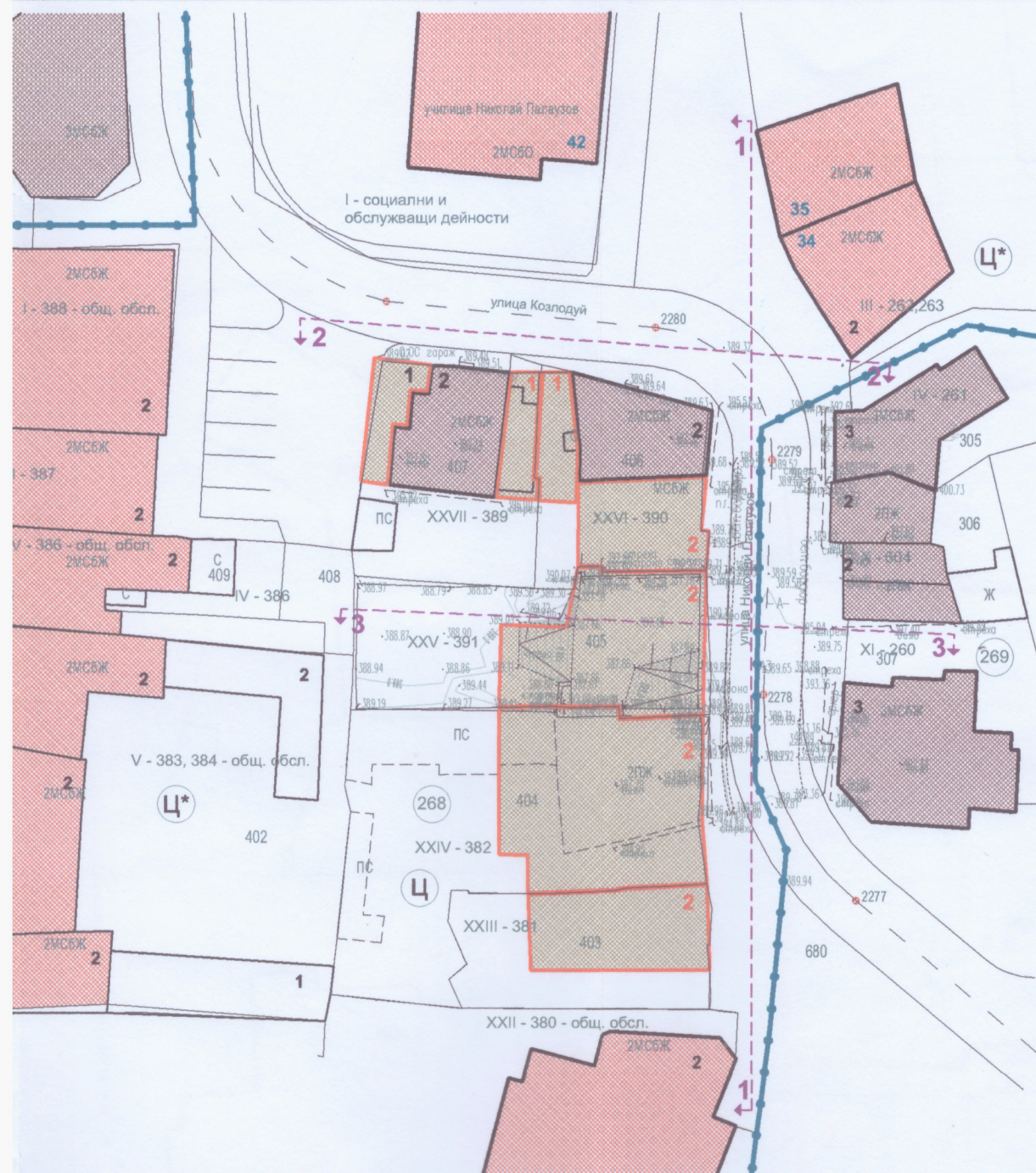
СИТУАЦИЯ М 1 : 500
