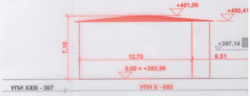
СИЛУЕТ ОТ ЮГОИЗТОК М 1 : 200
