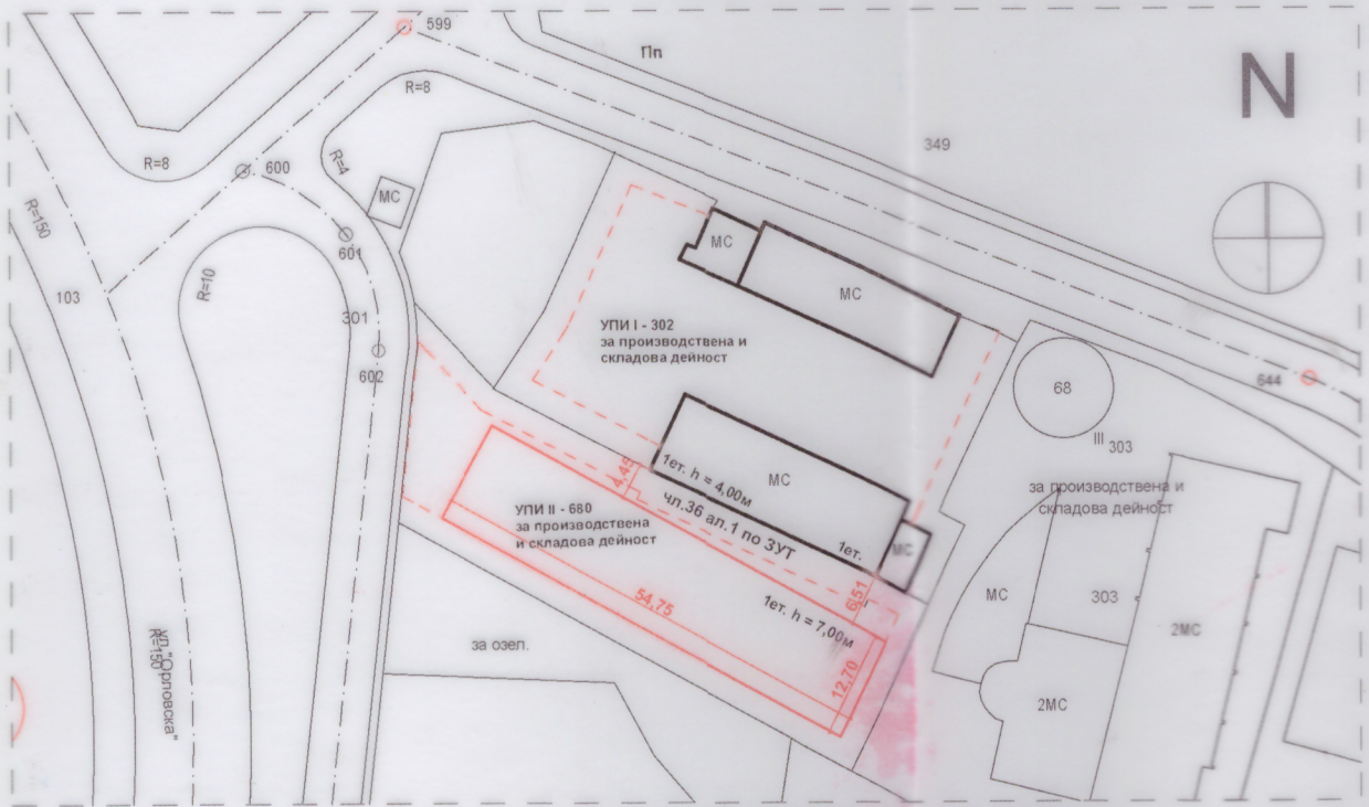
ПЛАН ЗА ЗАСТРОЯВАНЕ НА УПИ II - 680 ,КВ. 68 М 1 : 1000
