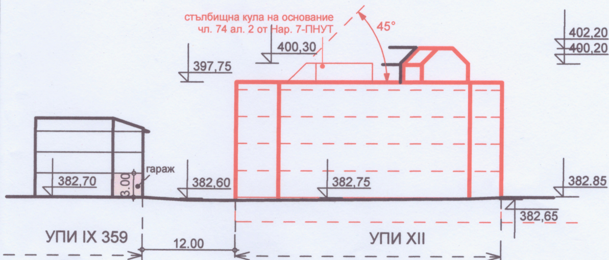
СИЛУЕТ 1-1 ПРЕЗ УЛИЦА ОТ 1250- 1250а М 1:500
