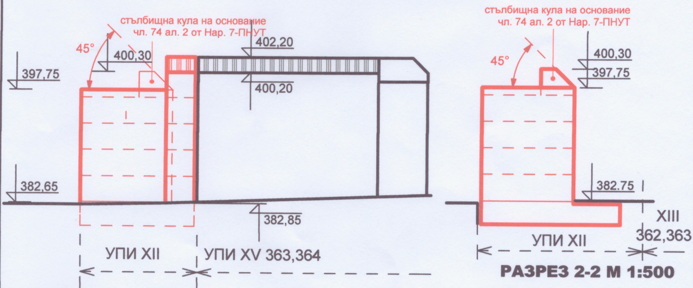
СИЛУЕТ ПО УЛИЦА ОТ 1429а- 2083 М 1:500
