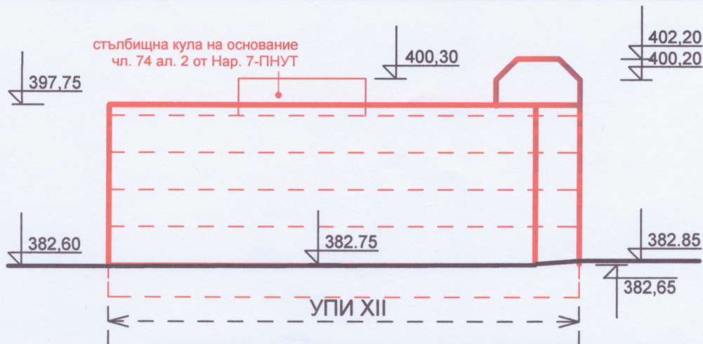
СИЛУЕТ ПО УЛИЦА ОТ 1250- 2083 М 1:500
