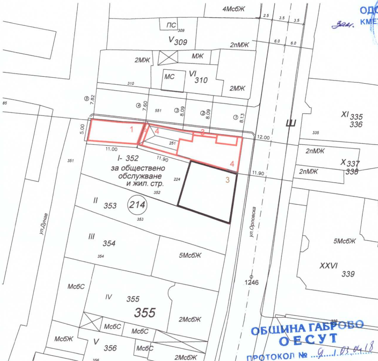
СИТУАЦИЯ М 1:500
